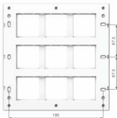
18 Module
