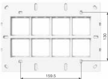
16 Module*
