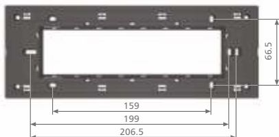
18 Module
