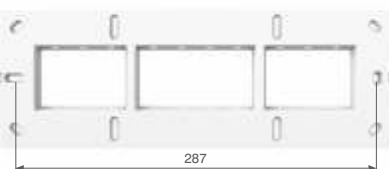
10 Module
