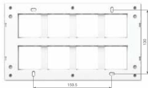
16 Module
