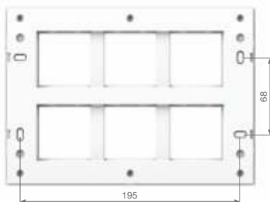
12 Module
