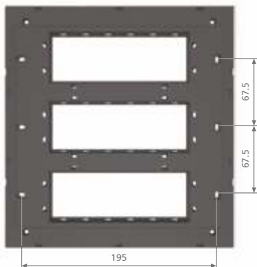
18 Module
