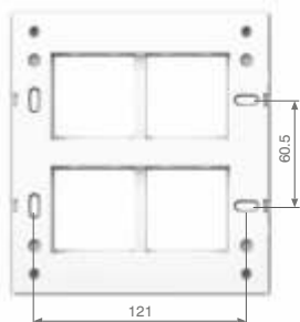
8 Module (V)
