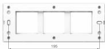
6 Module
