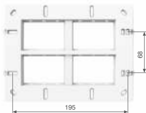
12 Module (V)*
