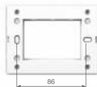
3 Module*
