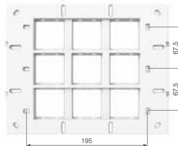
18 Module*
