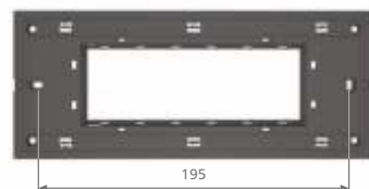
6 Module
